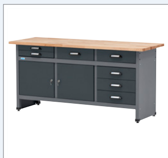
L 170 cm | H 84 cm | P 60 cm 2 portes verrouillables 5 tiroirs (H 12 cm) 2 tiroirs (H 6,5 cm) No art. 12278 (HB-Art. 12268090)
